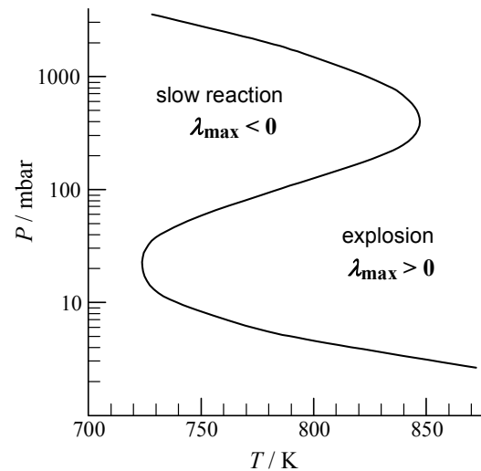
図 2.1: H 2 -O 2 爆発限界
