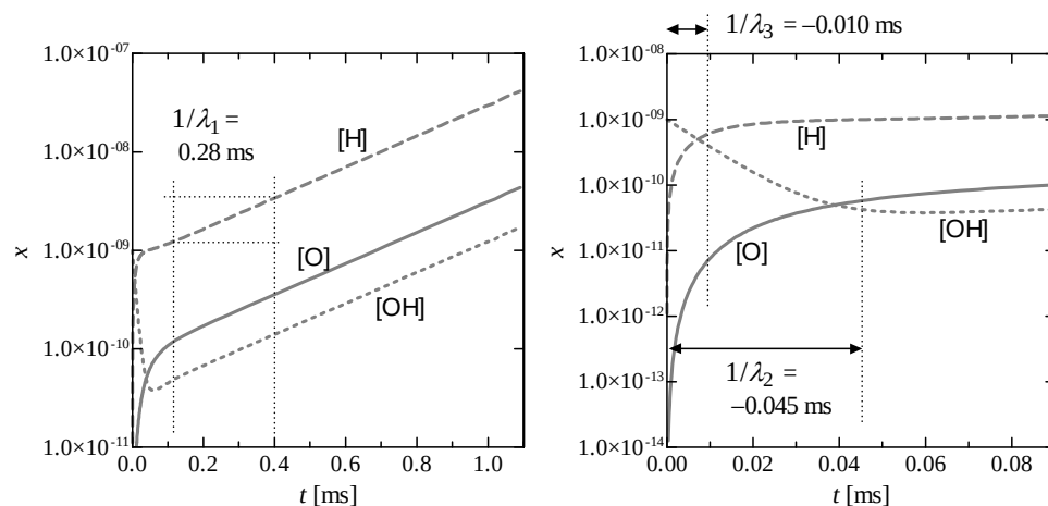
図 1.1: H 2 -O 2 連鎖反応
