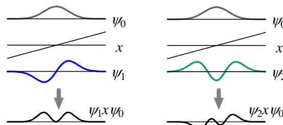
図 2.5a 許容遷移
