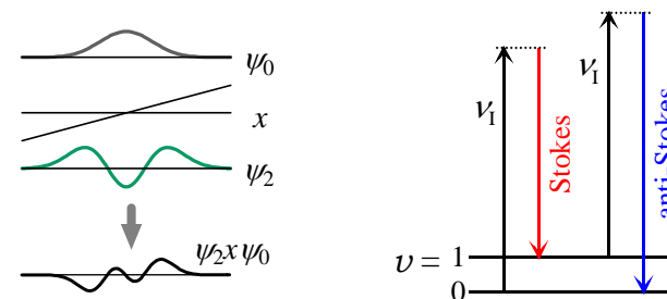
図 2.5b 禁制遷移
