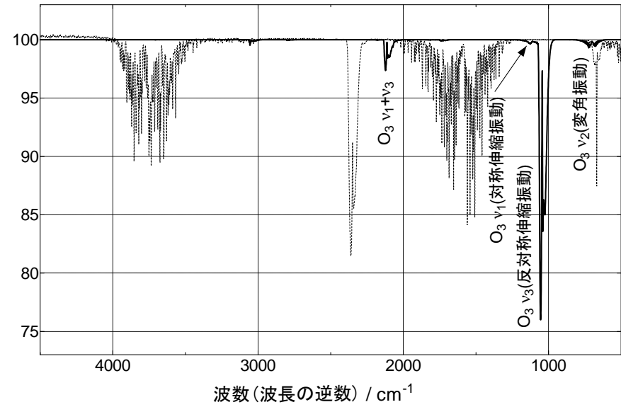
オゾン・大気赤外吸収スペクトル
