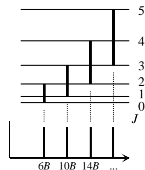
回転ラマン散乱スペクトル
