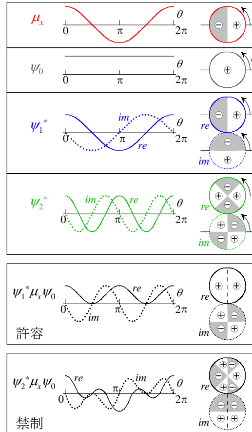
純回転遷移の選択則 (一次元回転子)
