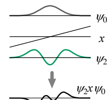
図 2.5b 禁制遷移
