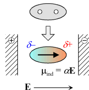
図 1.5 分極率と誘起双極子
