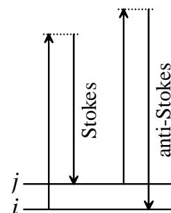
図 1.4 ラマン散乱
