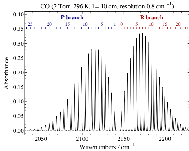
回転状態の ボルツマン分布
