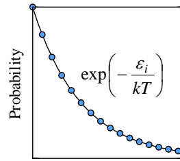
ボルツマン分布 (縮退のない場合)
