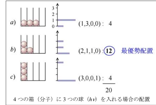
ボルツマン分布 – 統計力学的裏付
