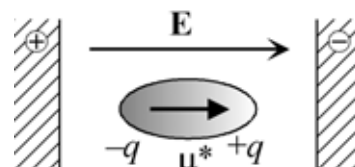
図 9.2 誘起双極子
