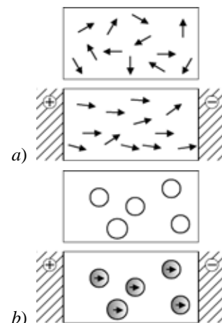
図 9.4 分極への
