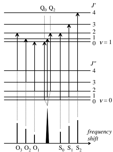
図 3.11 スペクトル枝 (Raman)
