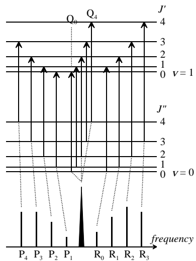
図 3.10 スペクトル枝 (IR)
