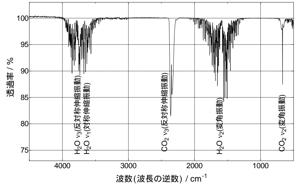
大気の赤外吸収スペクトル
